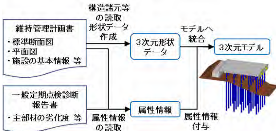
図-4 開発する3次元モデル簡易作成手法の概要
