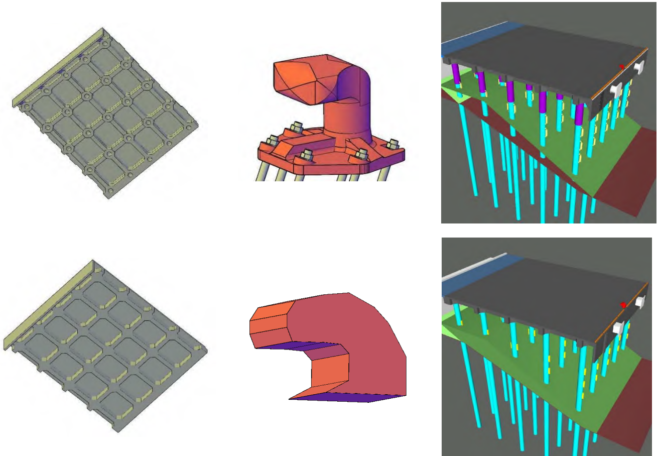
図-3 LoDの異なる3次元モデルの比較結果（上段：LoD300相当，下段：LoD200）
