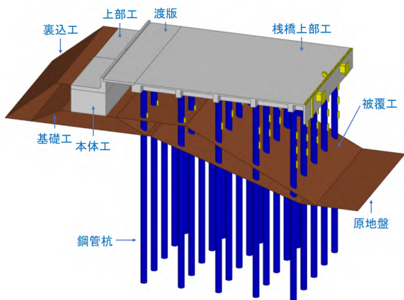
図-5 直杭式横栈橋の構成要素
