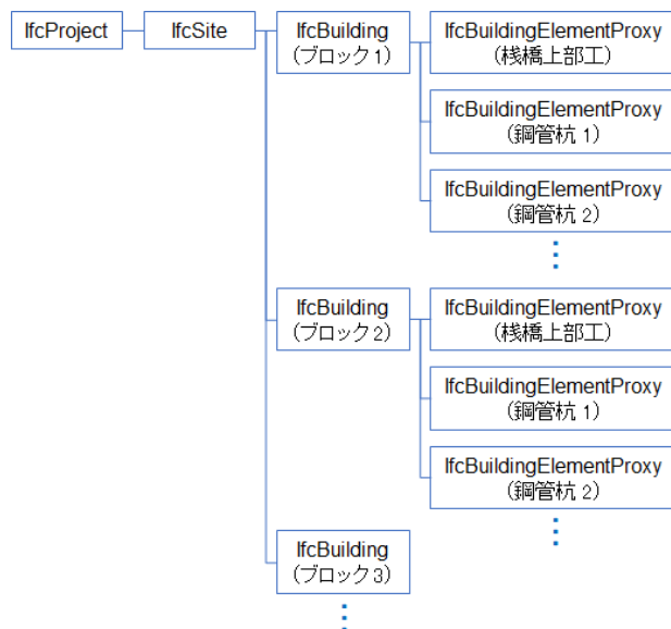
図-7 直杭式横栈橋の 3 次元モデルの IFC 形式のファイル構造
