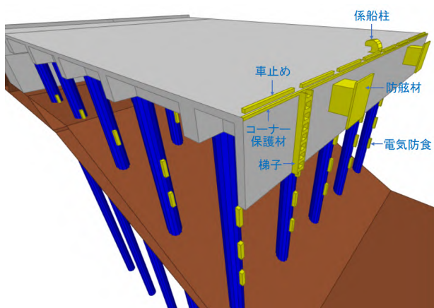
図-6 直杭式横栈橋の構成要素（付属工の拡大図）
